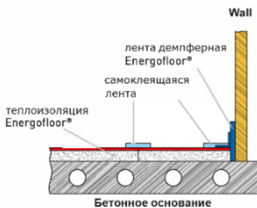
Схема установки тёплого пола
